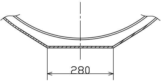
A・B部断面図
