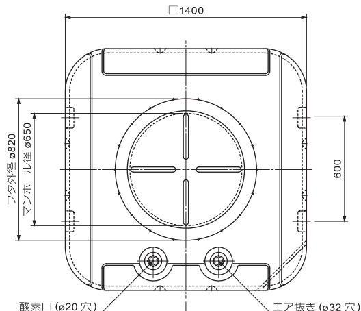
活魚タンク1000
